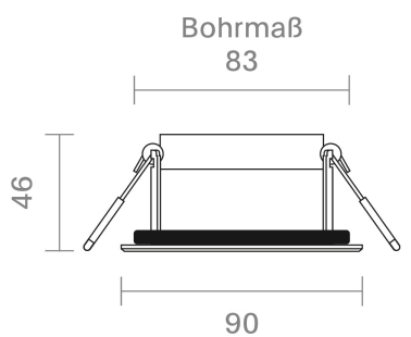
Einbauvariante mit Adapterring
